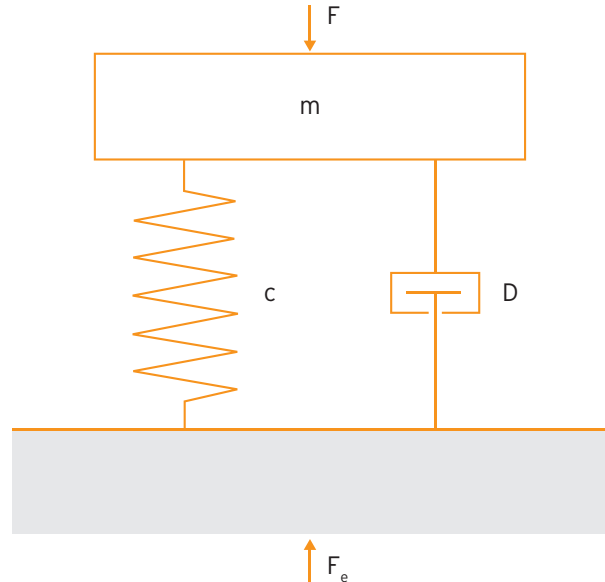
Abb. 8: Eindimensionales Masse-Feder-System
