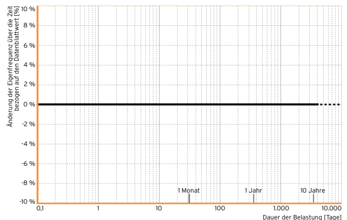
Abb. 7: Dynamisches Dauerstandverhalten von Sylomer®
