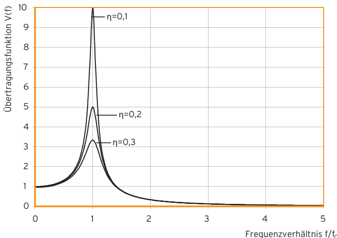
Abb. 10: Übertragungsfunktion
