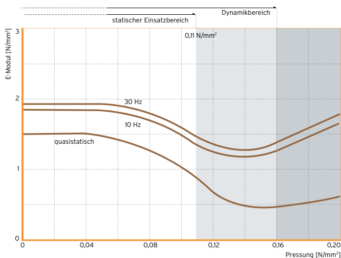
Abb. 3: Lastabhängigkeit des quasistatischen u. dynamischen E-Moduls am Beispiel Sylomer® SR110
