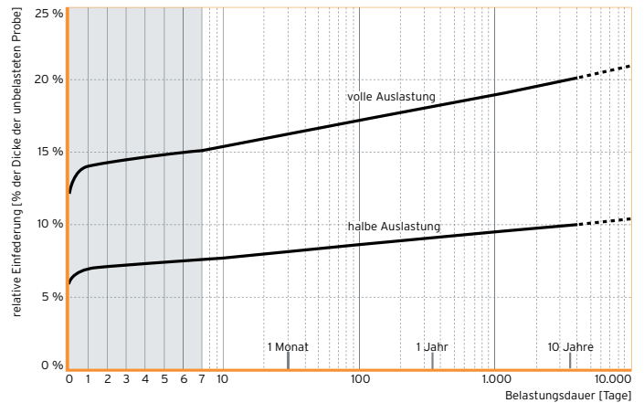
Abb. 6: Dauerstandverhalten von Sylomer®
