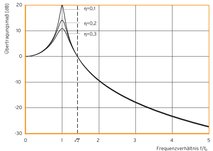
Abb. 11: Übertragungsmaß
