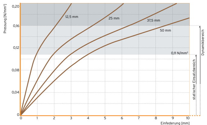
Abb. 2: Federkennlinien am Beispiel von Sylomer® SR110
