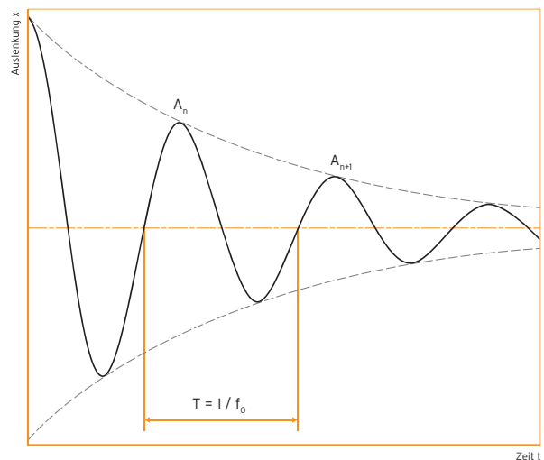
Abb. 9: Abklingverhalten einer freien Schwingung
