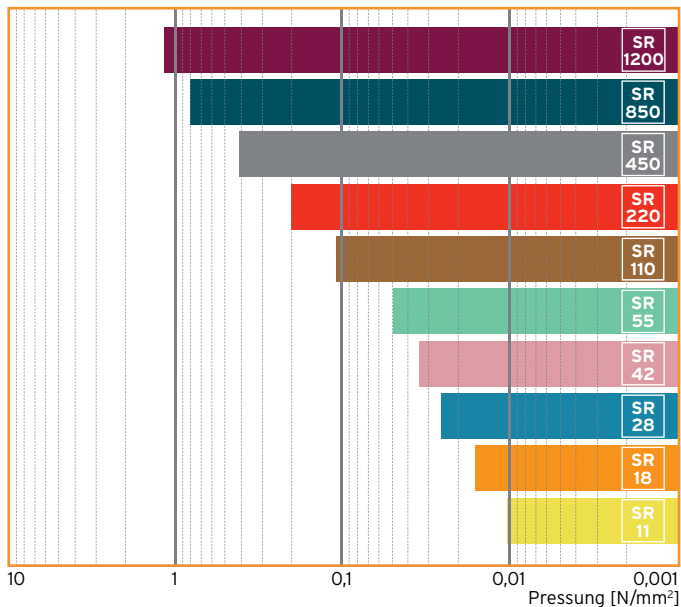
Abb. 1: Sylomer® Typenreihe
