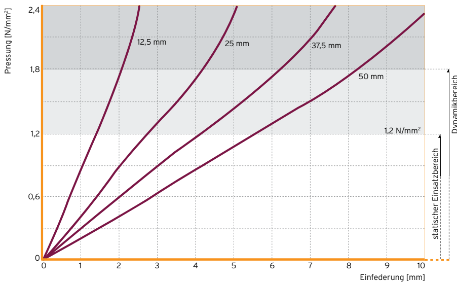
Abb. 1: Quasistatische Federkennlinie mit einer Belastungsgeschwindigkeit von 0,12 N/mm²/s
