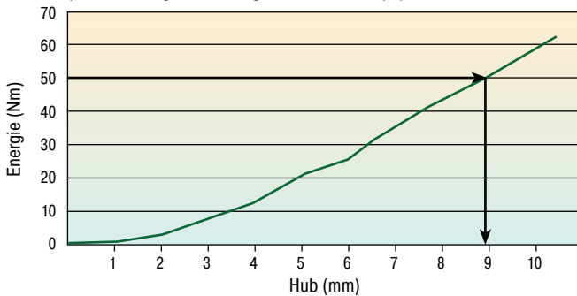
Energie-Hub Kennlinie (dynamisch) (bei Aufwahrgeschwindigkeit über 0,5 m/s)
