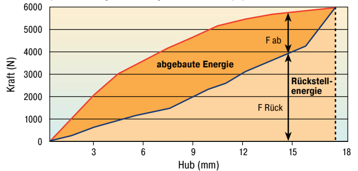
Kraft-Hub Kennlinie (dynamisch) (bei Aufwahrgeschwindigkeit über 0,5 m/s)
